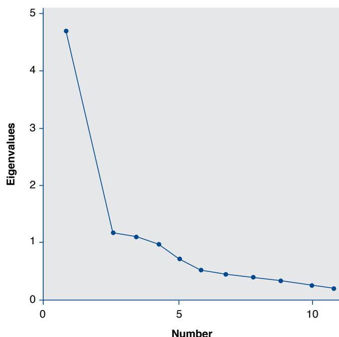
Figura 1. Gráfico de sedimentación para los autovalores del análisis factorial exploratorio de los 11 ítems de la escala IDA.
